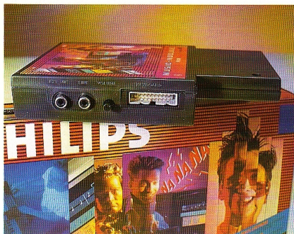
Sul lato sinistro del modulo, nell'ordine: la presa per un microfono esterno, la presa audio IN, la manopola del volume, ed il connettore per la tastiera sonora
