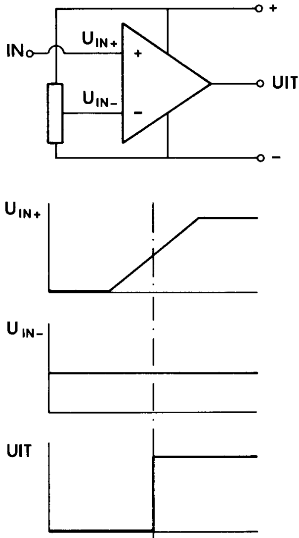
Afbeelding 19-6 Een eenvoudige vergelijkerschakeling.
