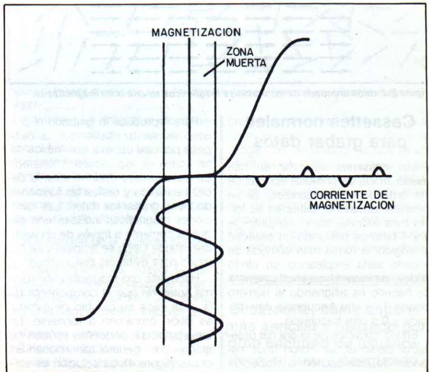
Figura 4: Sin polarización, el resultado es un grado elevado de distorsión.
