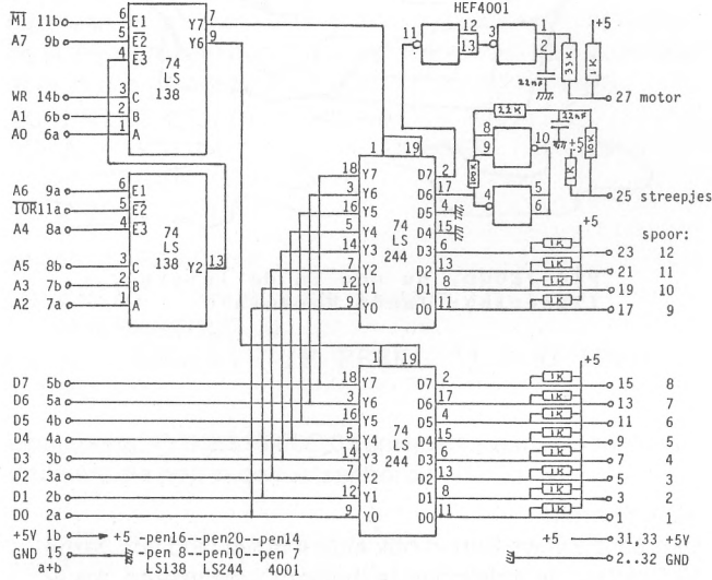
Figuur 1: schema van de interface voor de aansluiting van de MR-500 op de P2000.
