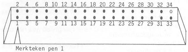
Figuur 3: nummering van de 34-polige-connector.
