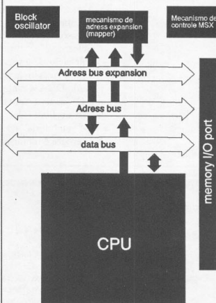
Figura 5 - Esquema do R800 CPU
