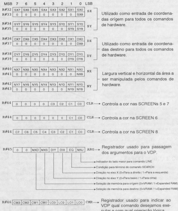
FIGURA 2 – Registradores utilizados pelos comandos de hardware
