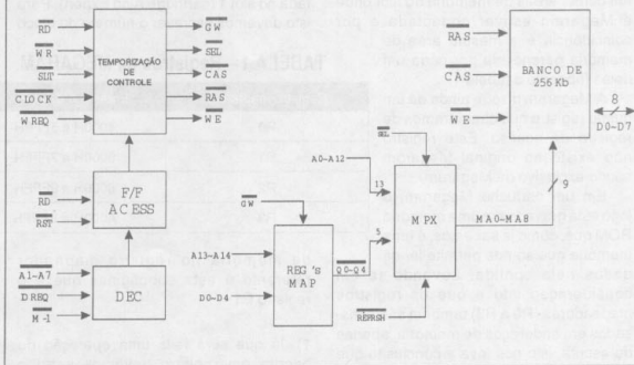
FIGURA 2 - Diagrama em blocos da Megaram (256 Kb)
