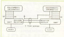
Ligação Assíncrona Típica
