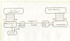
Ligação Síncrona Típica
