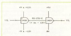
Efetivação de uma ligação RS-232-C com os componentes clássicos 1488 e 1489
