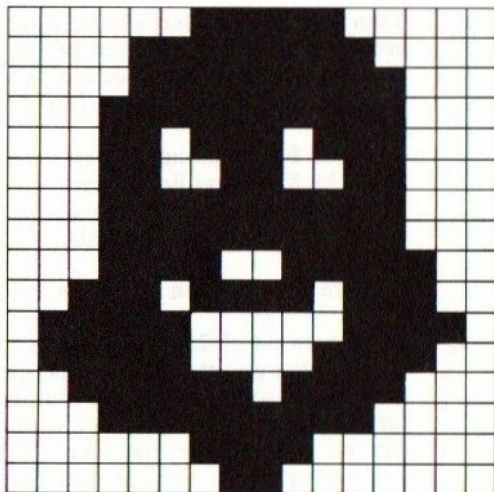
16x16 sprite
