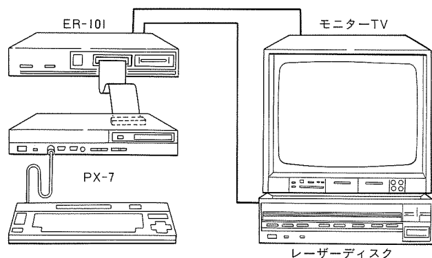
図9.1 接続
