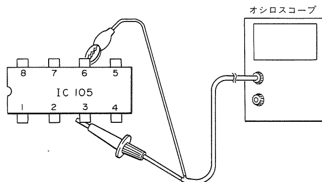
図9.3 同期分離調整
