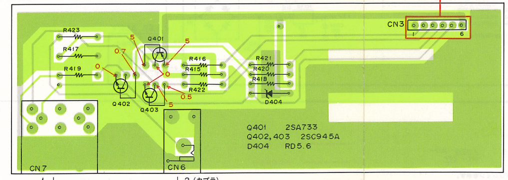
システムコントロールAss'y (R974105B)
