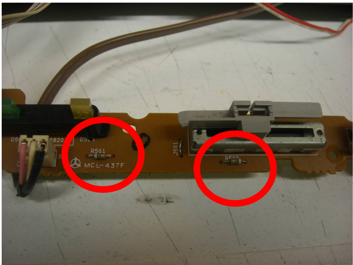
Frontprint voor de wijziging
