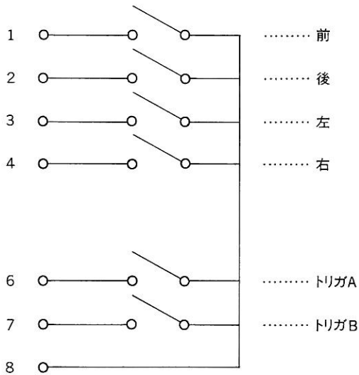
図 1.13 ジョイスティック回路接続図
