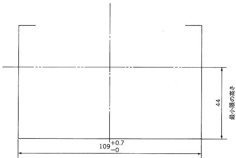
図 1.32 コネクタ例
