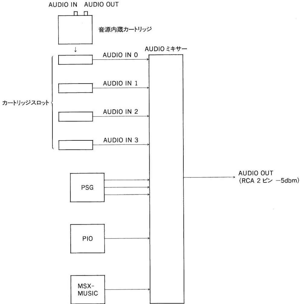
図 1.9 MSX の音声出力
