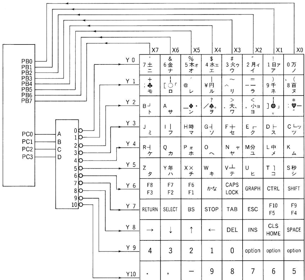
図 1.6 キーのマトリックス
