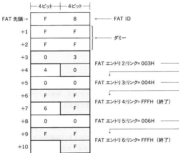
図 3.17 FAT の実例
