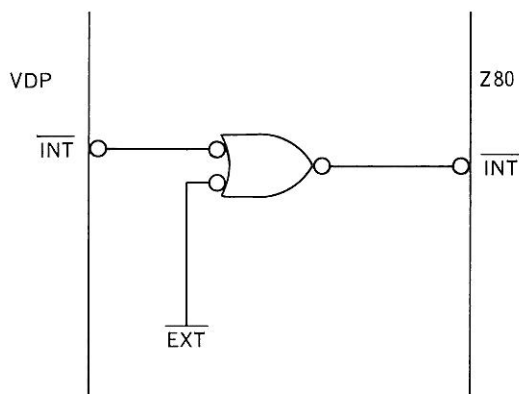
図 1.4 割り込み回路例
