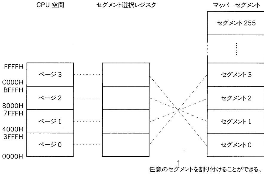
図 1.1 メモリマッパーの論理的構成
