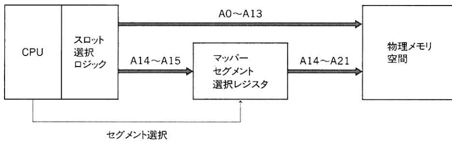
図 1.2 メモリマッパーの物理的構成
