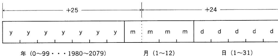
図 3.22 日付を表すビットフィールド
